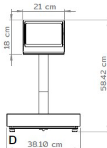
Vista frontall
